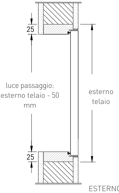
VISTA IN SEZIONE
