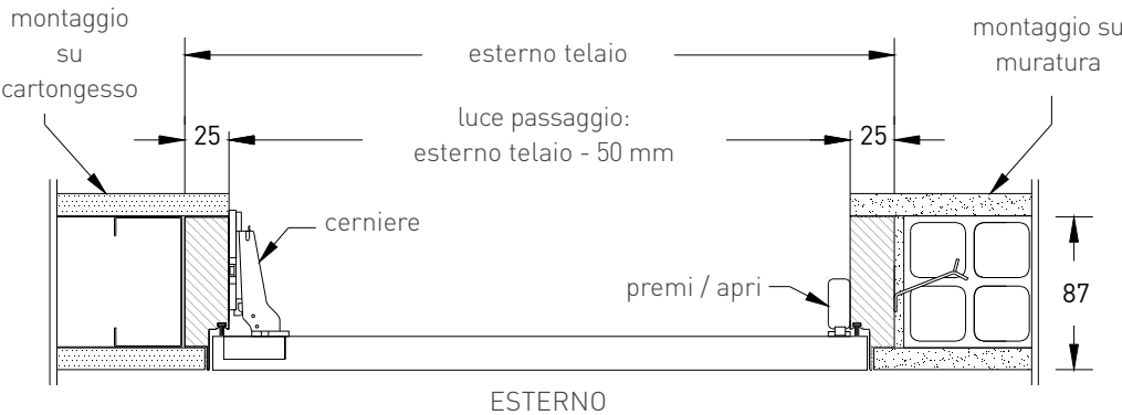
VISTA IN PIANTA
