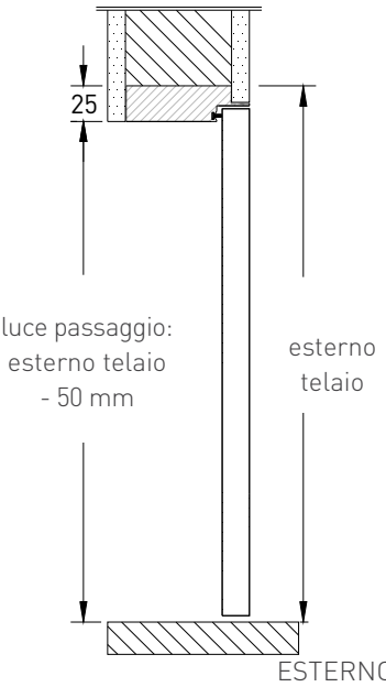
VISTA IN SEZIONE
