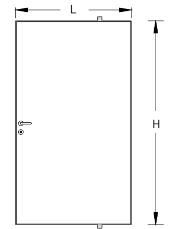
TAILOR-MADE DOOR
